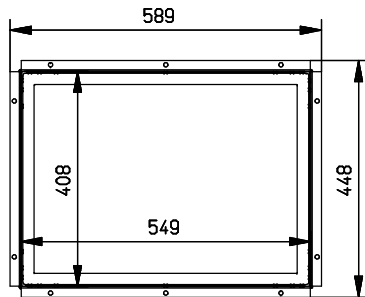
Einbaurahmen
