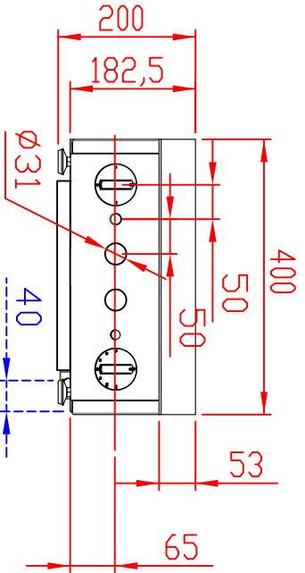
Vorderansicht
