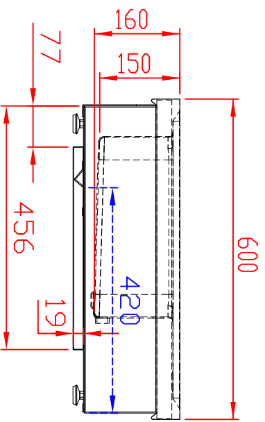
Seitenansicht
