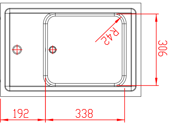
Draufsicht
