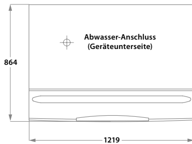
Draufsicht
