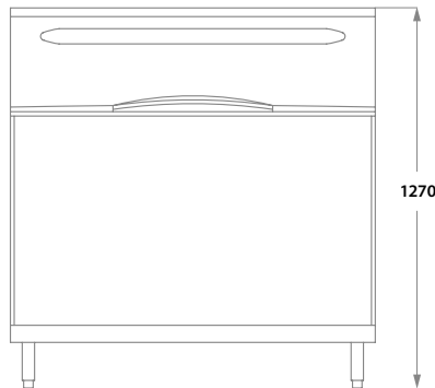
Frontansicht
