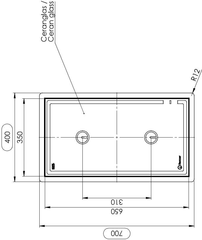
Draufsicht / Top view Variante A / Version A
