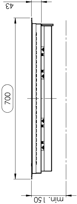
Seitenansicht / Side view Variante A / Version A
