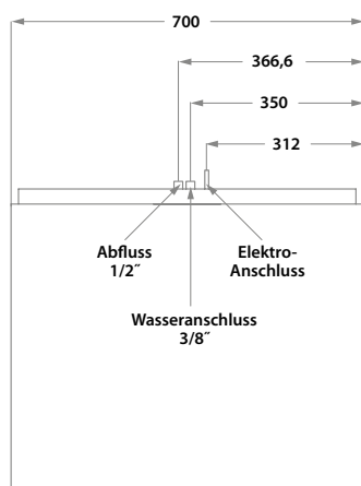
Draufsicht
