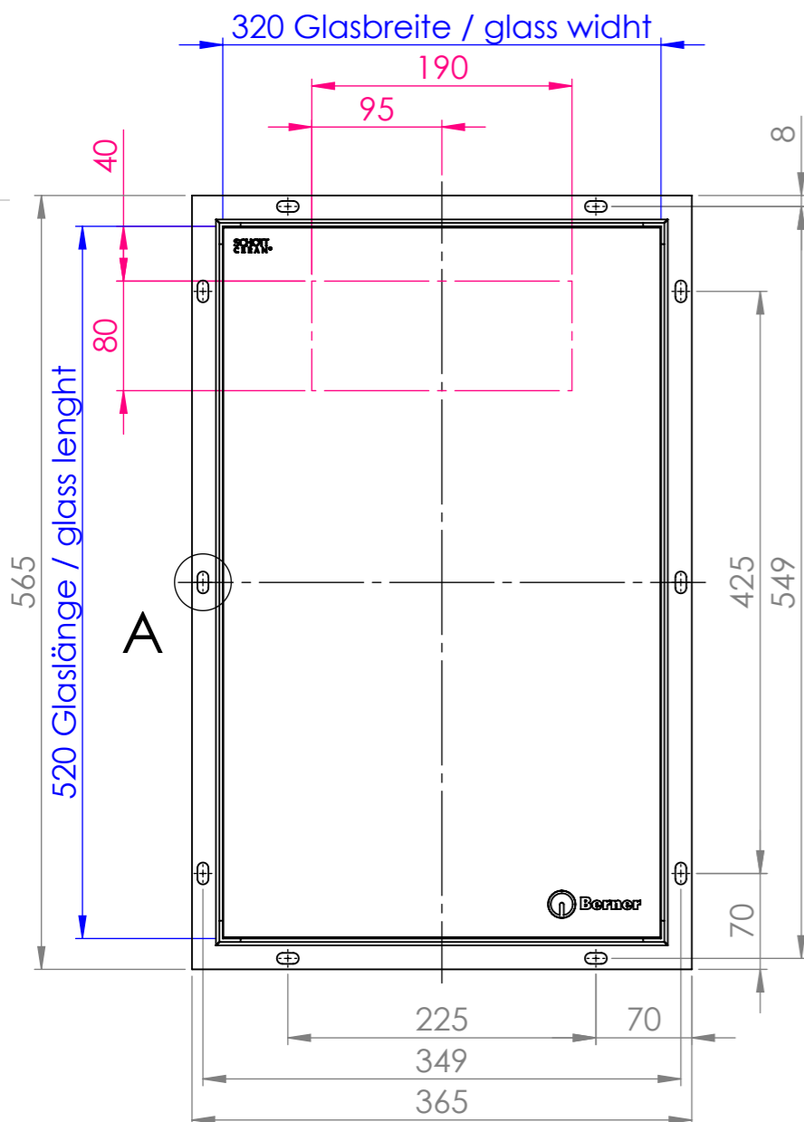
Draufsicht / top view
