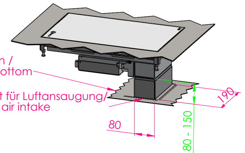
Lüfterausschnitt / Cut out for air intake
