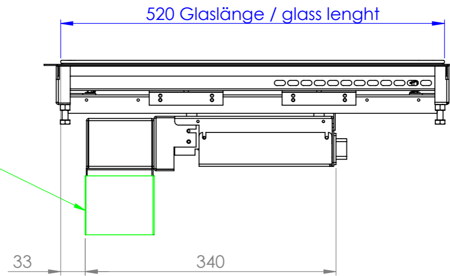
Lüfterausschnitt / Cut out for air intake
