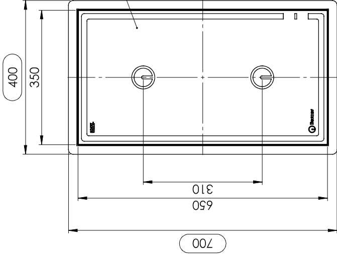
Draufsicht / Top view Variante A / Version A
