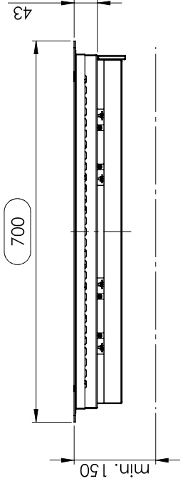
Seitenansicht / Side view Variante A / Version A
