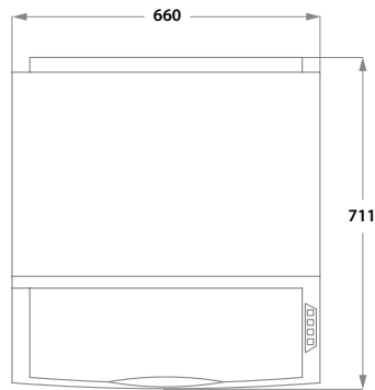
Draufsicht
