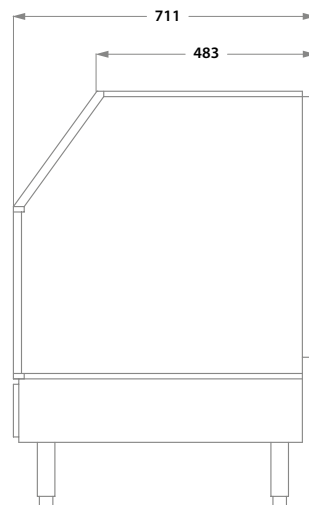
Seitenansicht
