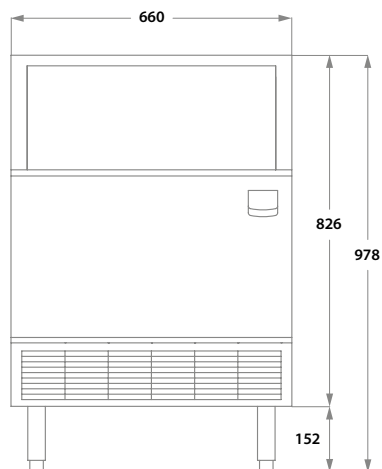
Frontansicht
