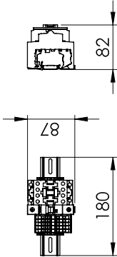
Schaltung / circuit :
